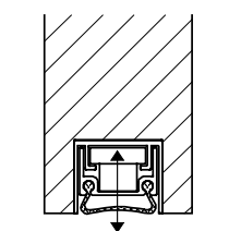
Absenkndichtung
